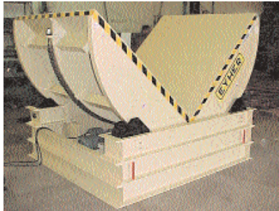
① Volteadores de 90° para moldes, palets, contenedores con botellas, etc. 0,5 a 60 t.
